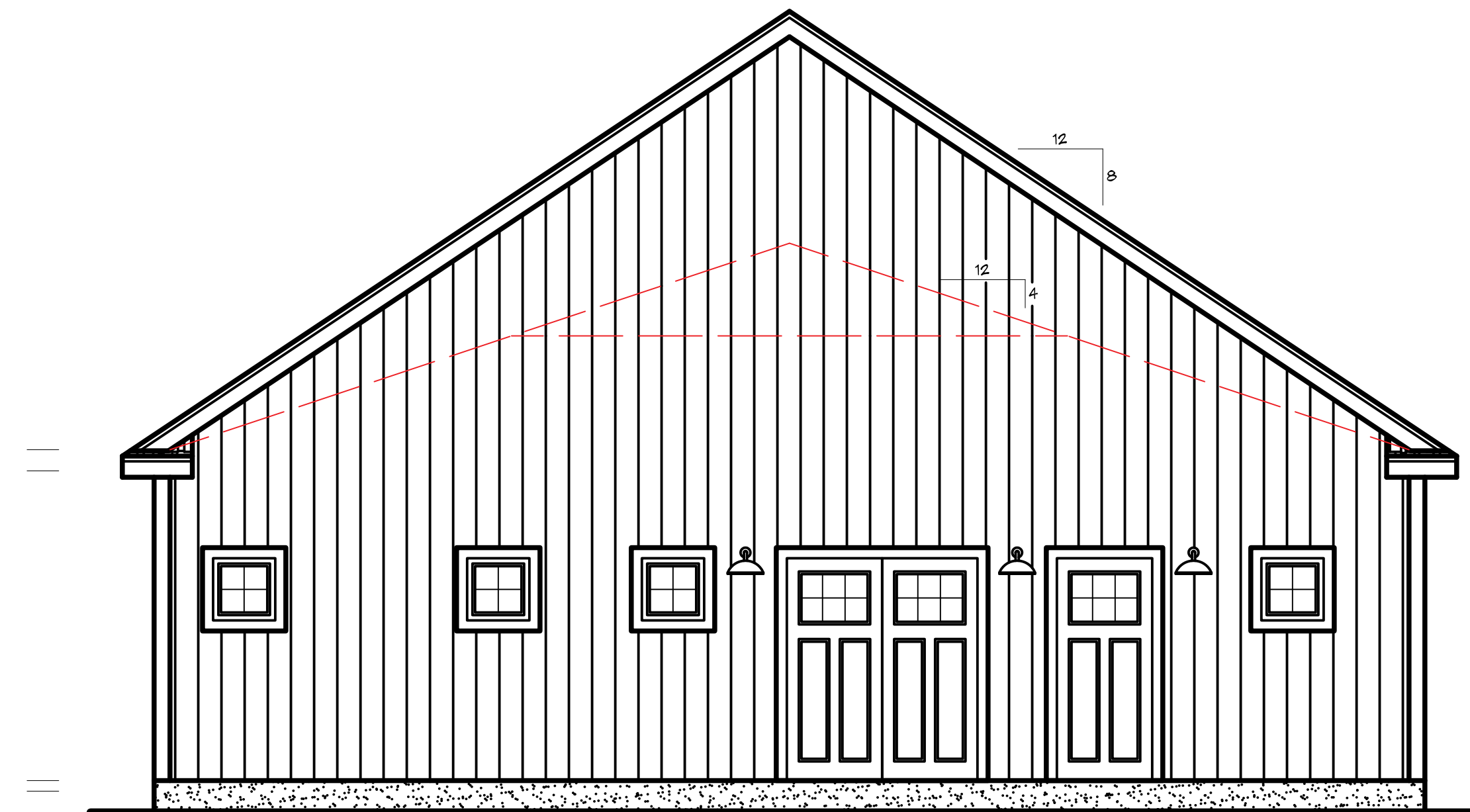
RIGHT ELEVATION
